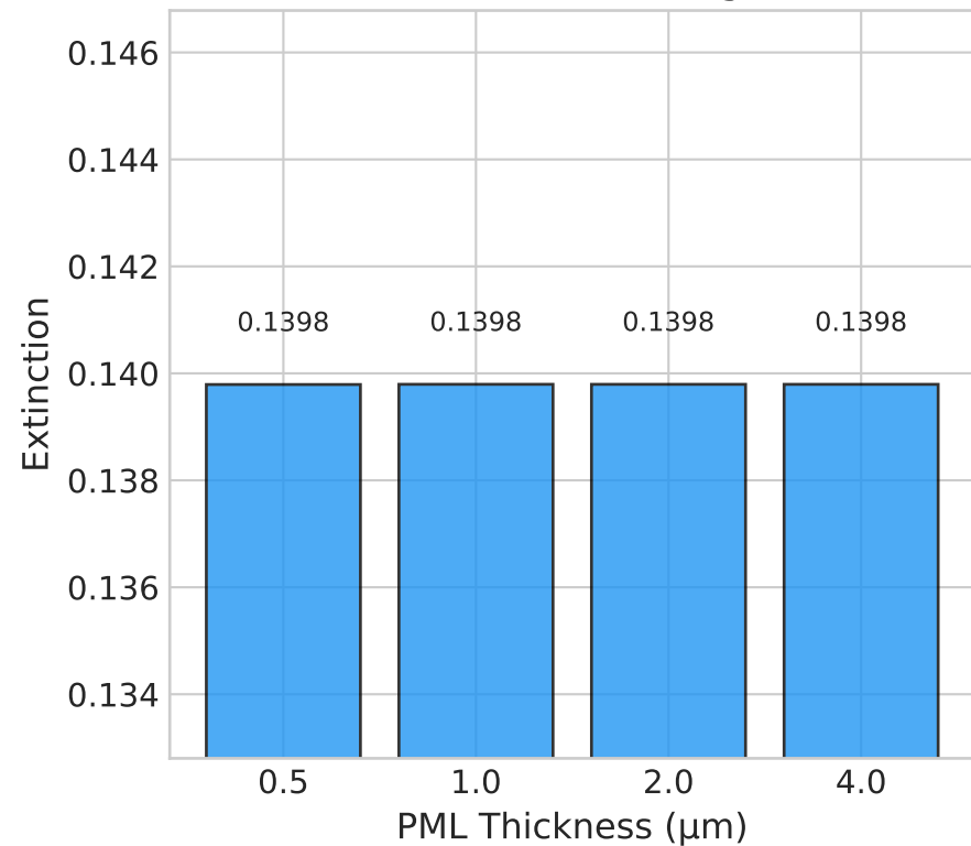
(a) Mie Scattering
