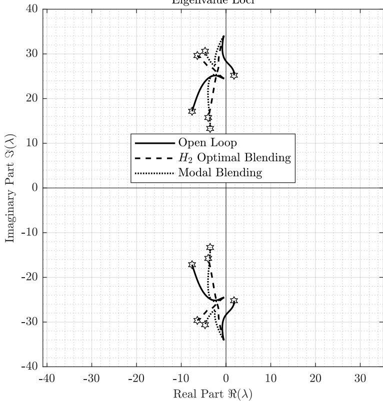
Eigenvalue Loci
