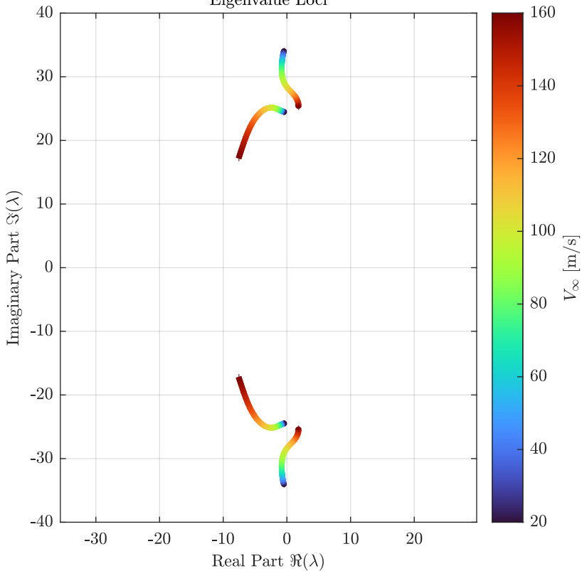
Eigenvalue Loci
