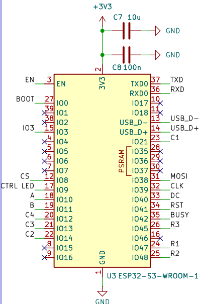
ESP32
