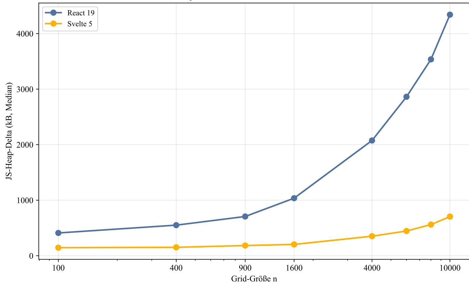
H3: Speicherverbrauch nach GC bei f = 10 Hz
