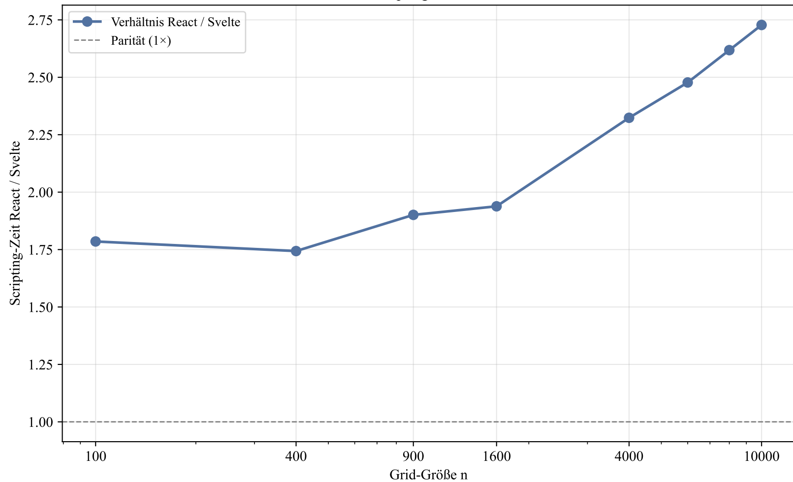
H2: Wachstum des Scripting-Overheads relativ zu Svelte
