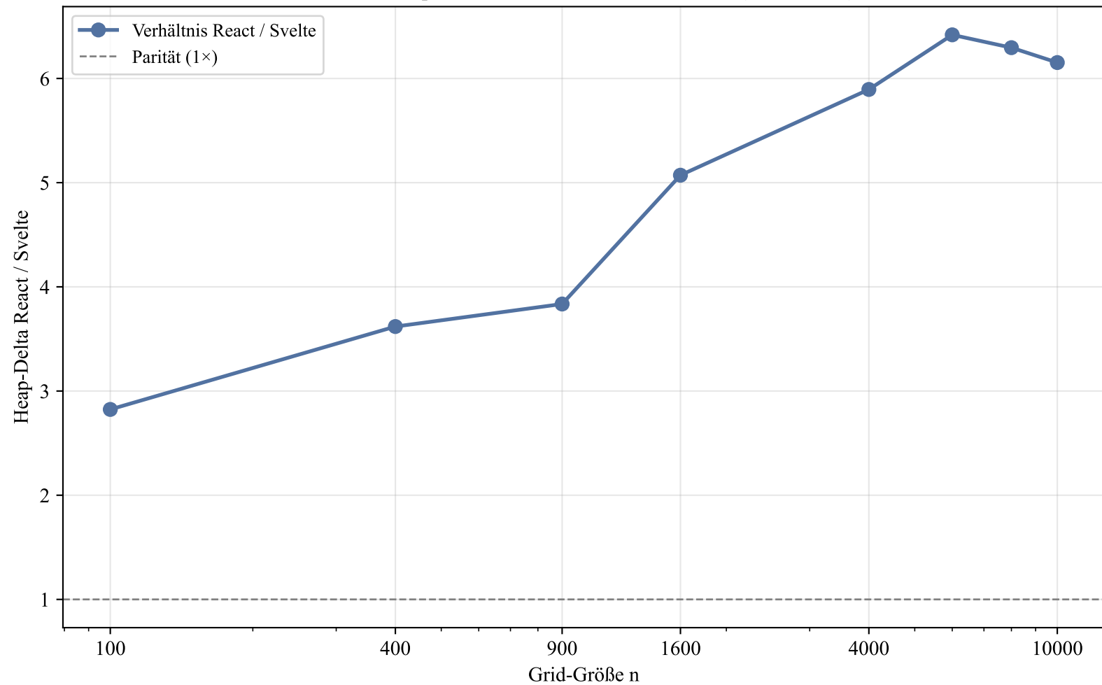
H3: React-Speicher-Overhead relativ zu Svelte (3× bis 6,4×)
