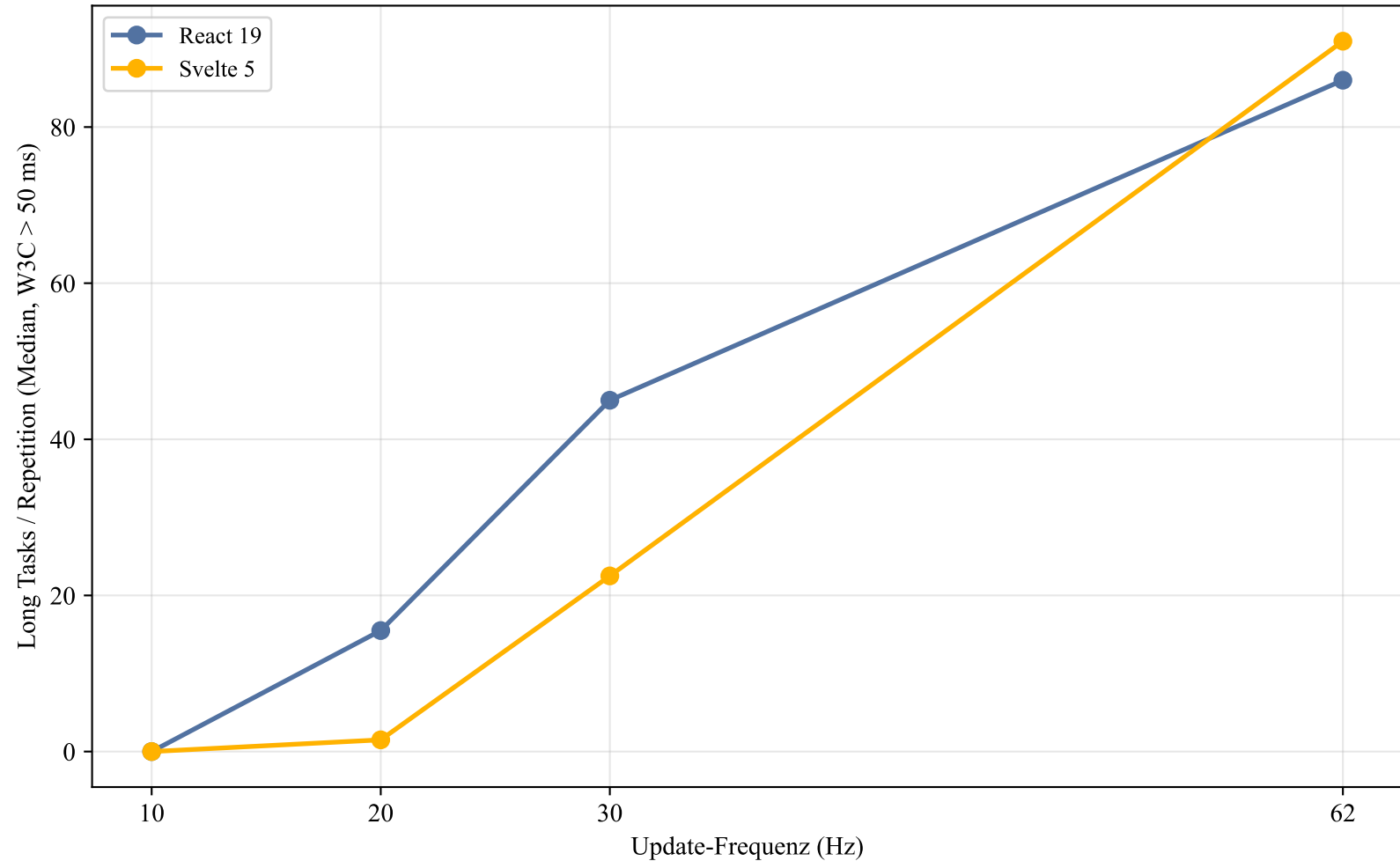
H4: Long Tasks bei n = 10.000 — Kreuzungspunkt
