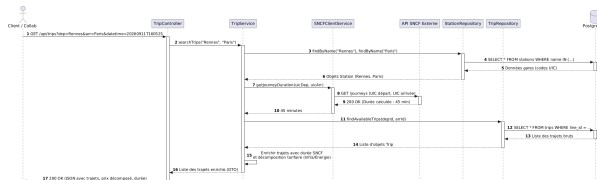
FIGURE 2.4 – Diagramme de séquence
