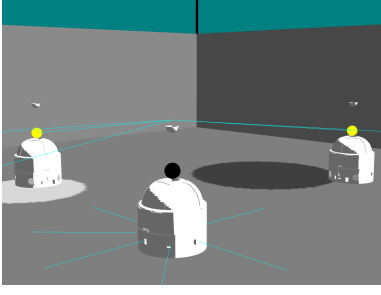
Fig. 1. Vista del modelo del robot QUPA implementado en ARGoS3. La plataforma está equipada con sensores infrarrojos para la percepción local y LEDs direccionales para la emisión de señales visuales.
