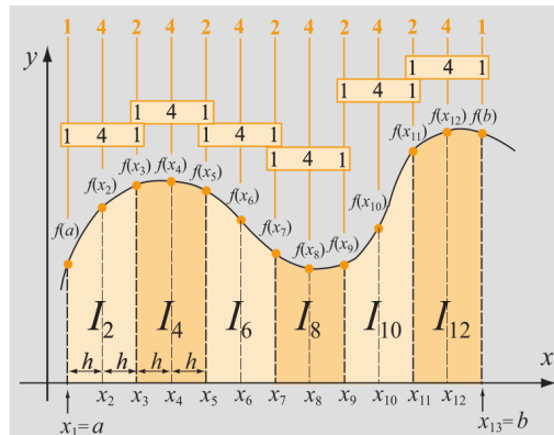
Figura 13: Regra de Simpson 1/3 composto
