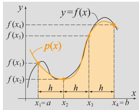
Figura 14: Regra de Simpson 3/8
