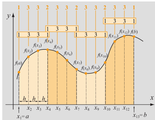
Figura 15: Aplicação sucessiva da regra 3/8
