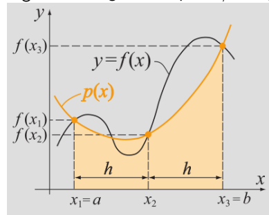
Figura 12: Regra de Simpson 1/3 Simples.
