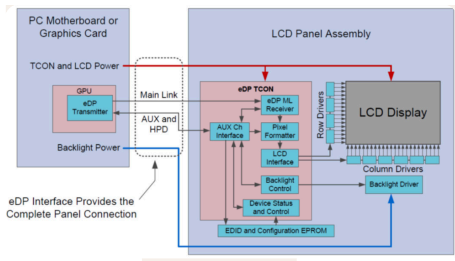
Fig. 6.35: TCON
