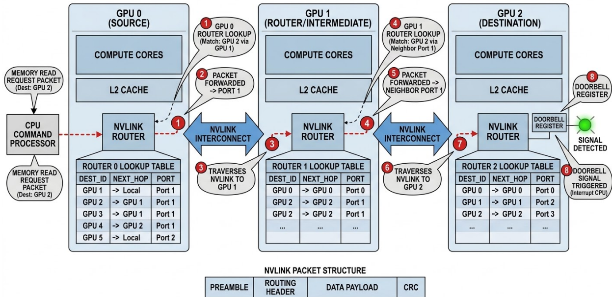
Fig. 6.36: NVLINK
