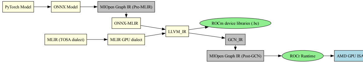
Fig. 2.93: AMD IR Conversion Flow
