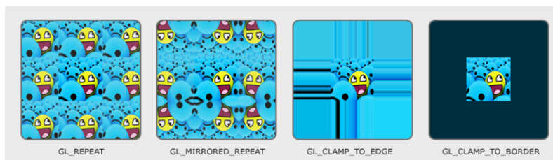
Fig. 2.81: Texture Warpping
