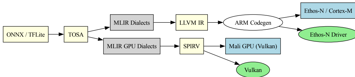
Fig. 2.94: ARM IR Conversion Flow
