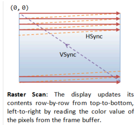
Fig. 3.8: VSync 10
