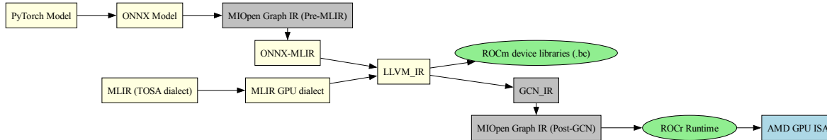
Fig. 7.8: AMD IR Conversion Flow
