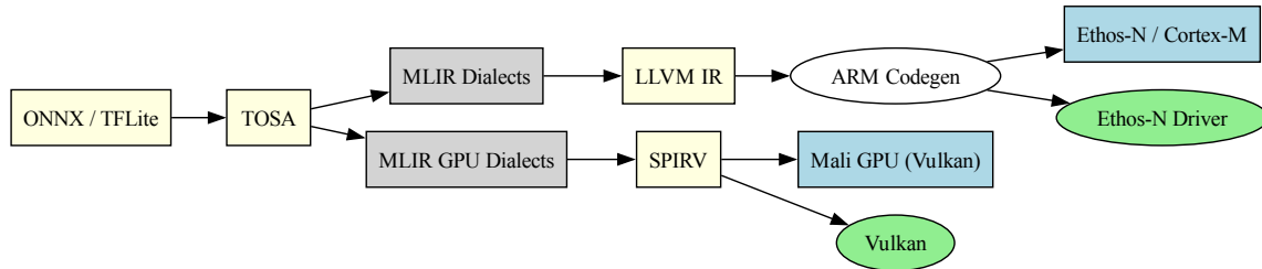
Fig. 7.10: ARM IR Conversion Flow
