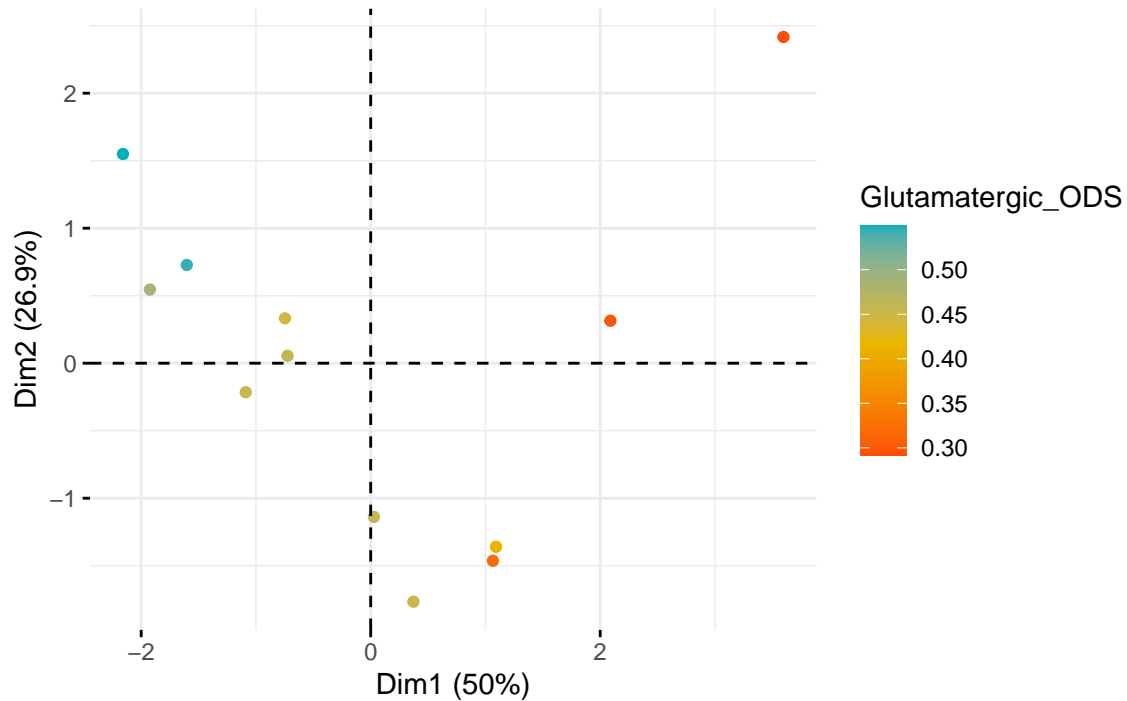
Individuals – PCA
