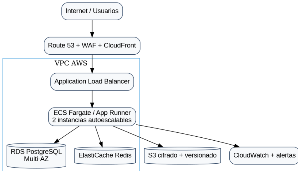
Figura 2. Despliegue simplificado en AWS.
