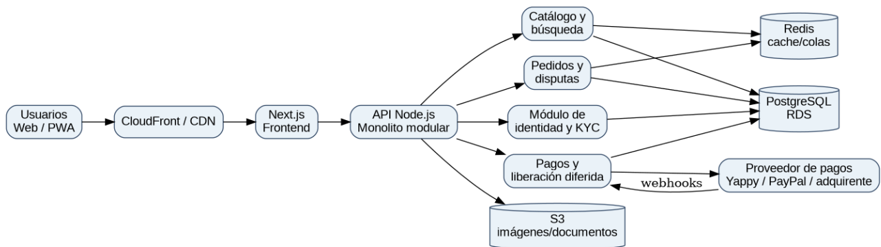
Figura 1. Arquitectura lógica propuesta para el MVP.
