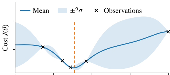
(a) Gaussian process posterior
