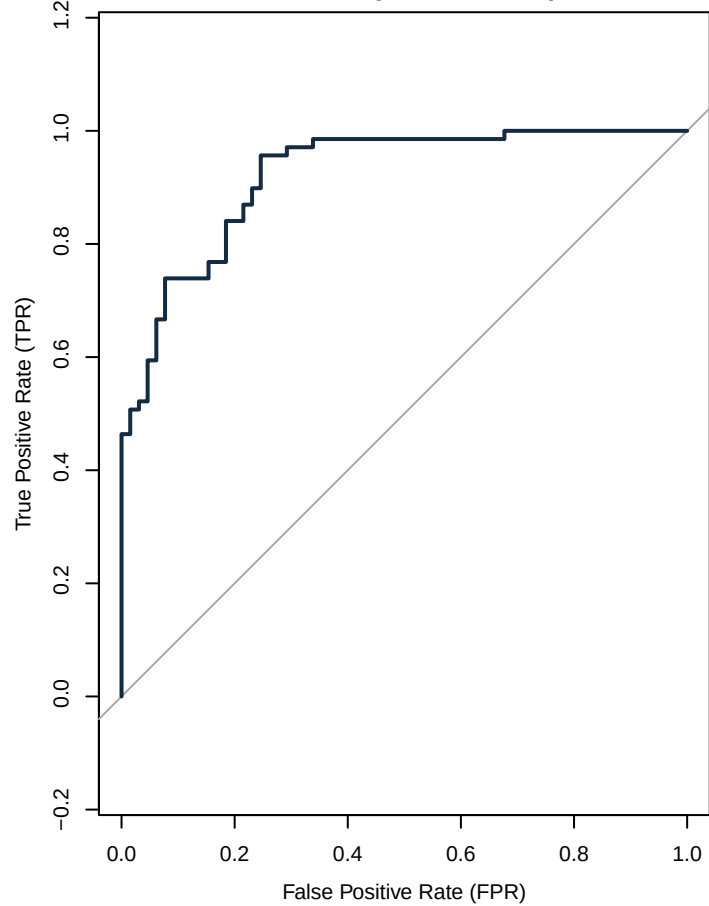
XGBoost (AUC = 0.9215)
