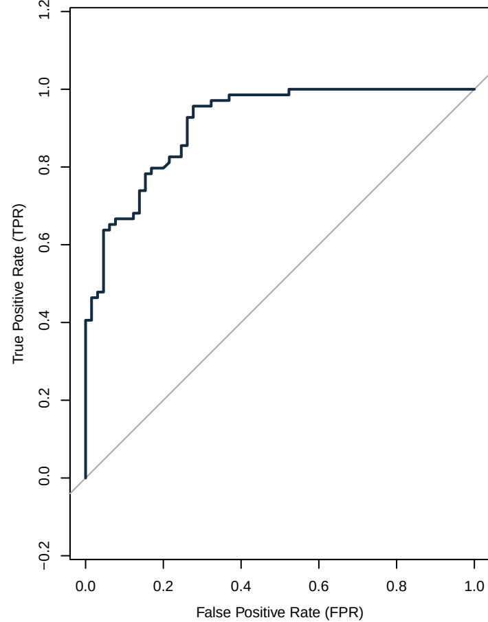
Monte Carlo (AUC = 0.9125)
