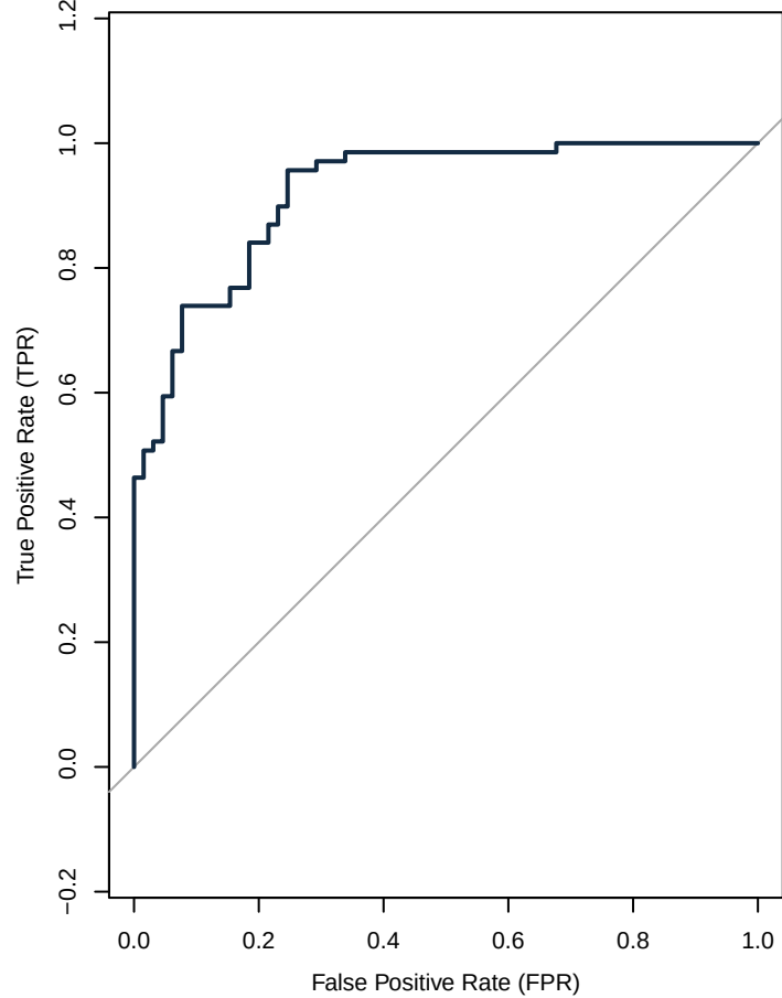
XGBoost (AUC = 0.9215)
