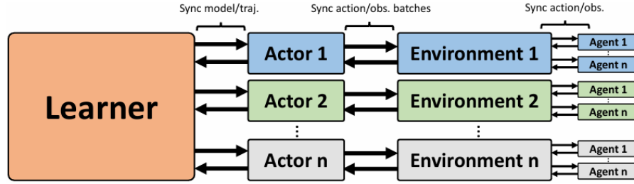
图 2-2: 系统架构
