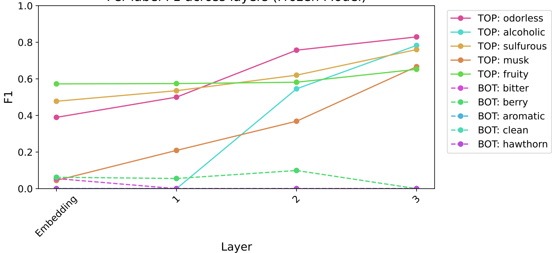
Per-label F1 across layers (Frozen Model)
