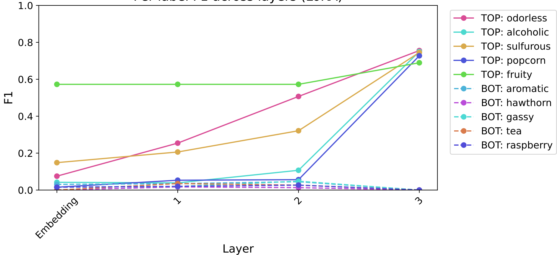
Per-label F1 across layers (LoRA)
