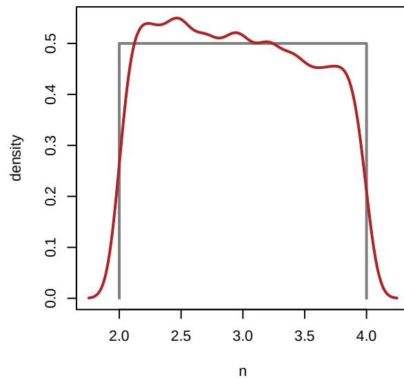
CESM2-WACCM - n
