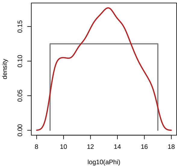
CESM2-WACCM - aPhi
