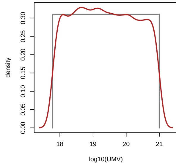
MIROC-ES2L - UMV
