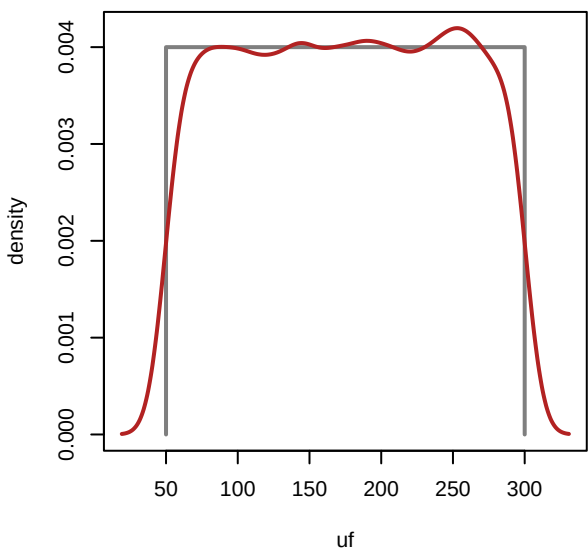
MRI-ESM2-0 - uf
