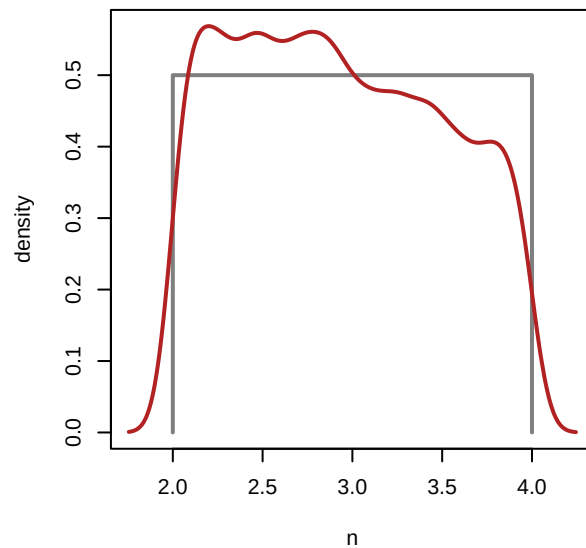
EC-Earth3-Veg - n
