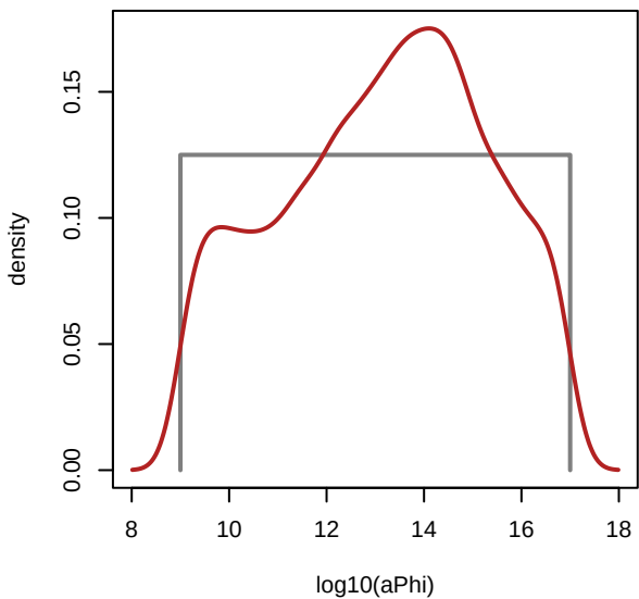
EC-Earth3-Veg - aPhi
