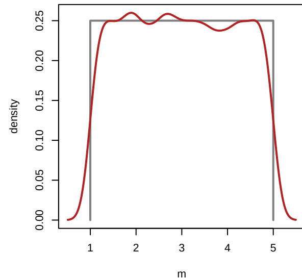
MIROC-ES2L - m
