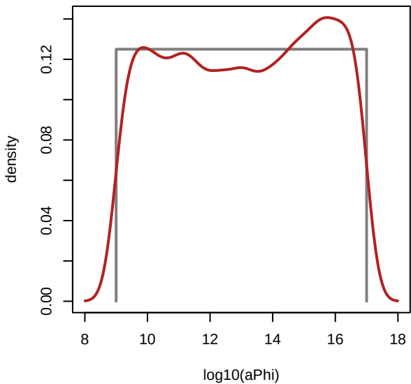
MIROC-ES2L - aPhi
