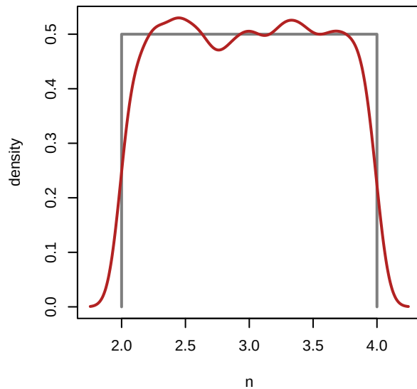
MIROC-ES2L - n
