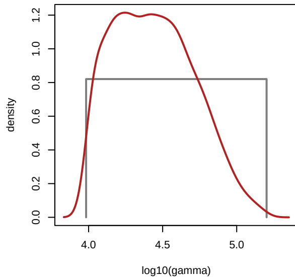
MIROC-ES2L - gamma
