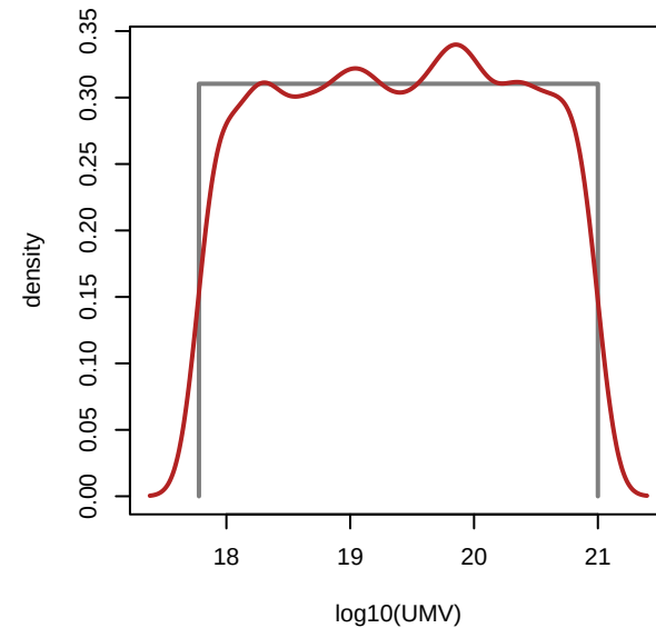
EC-Earth3-Veg - UMV
