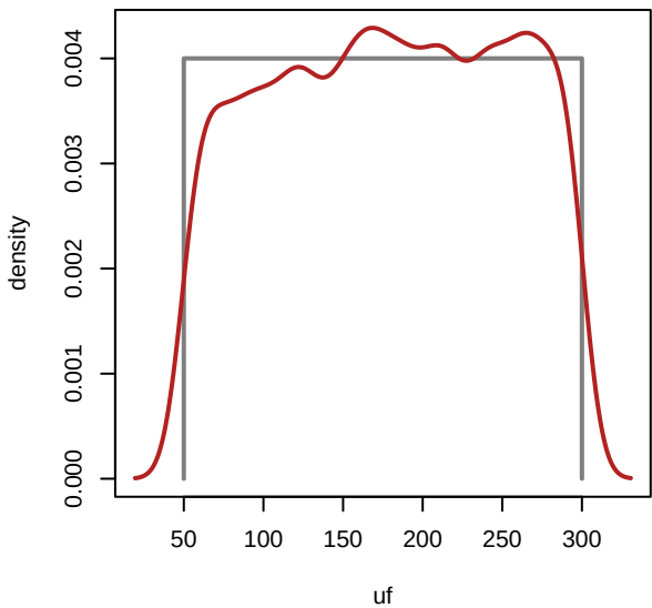
MIROC-ES2L - uf
