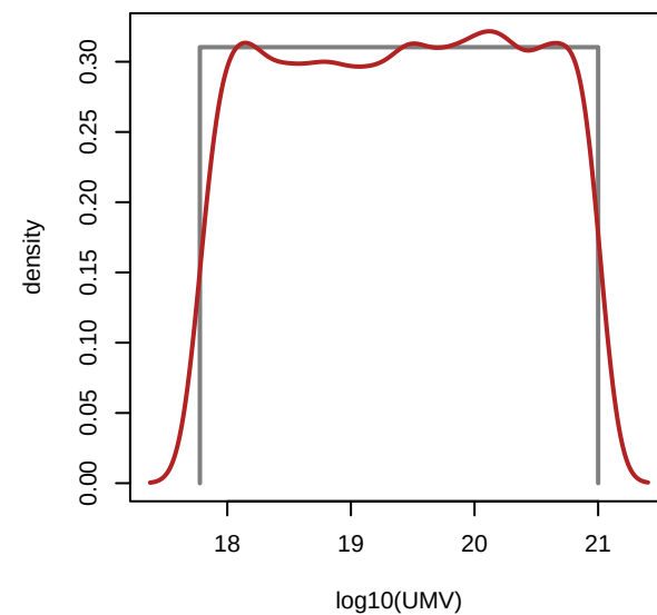
CESM2-WACCM - UMV
