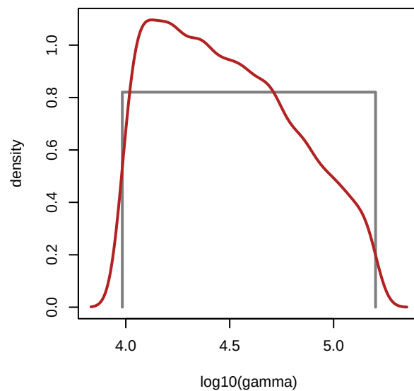
CESM2-WACCM - gamma
