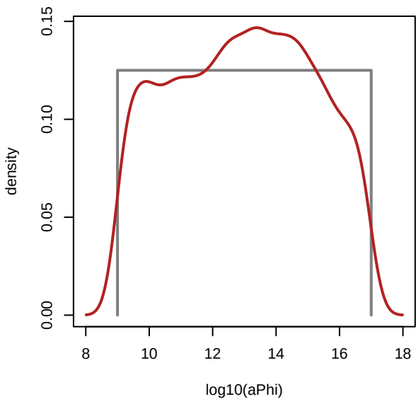
MRI-ESM2-0 - aPhi
