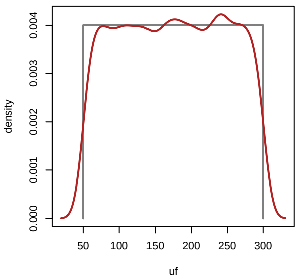
CESM2-WACCM - uf
