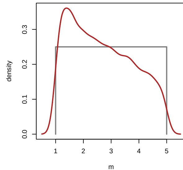
EC-Earth3-Veg - m
