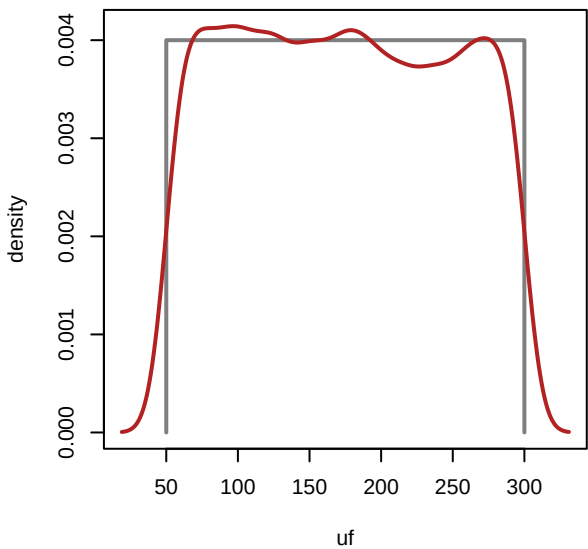
EC-Earth3-Veg - uf
