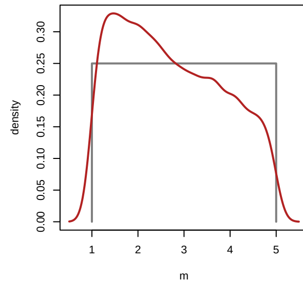
CESM2-WACCM - m
