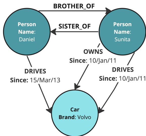
Abbildung 2.3: Labeled Property Graph
