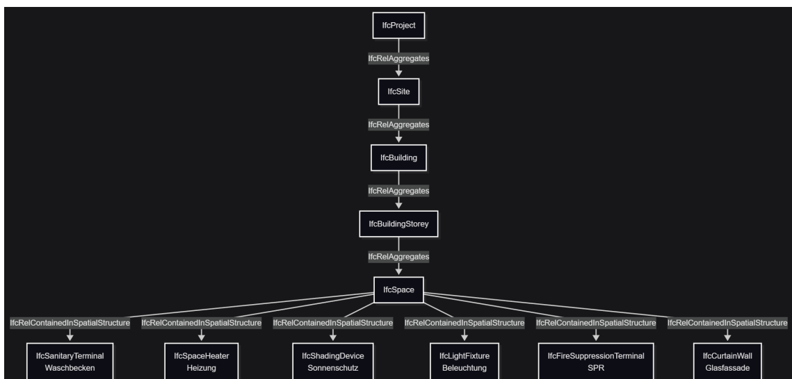
Abbildung 2.2: Struktureller Aufbau der IFC-Klassen.
