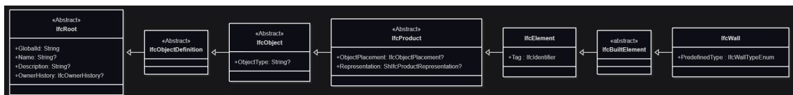
Abbildung 2.1: Hierarchischer Aufbau der IFC-Klassen.
