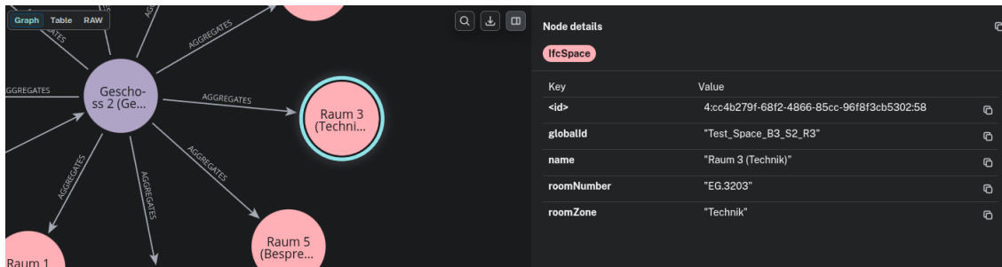
Abbildung 3.1: Beispiel für die Speicherung von Attributen in Knoten im Neo4j Browser
