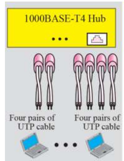
d. 1000BASE-T4
