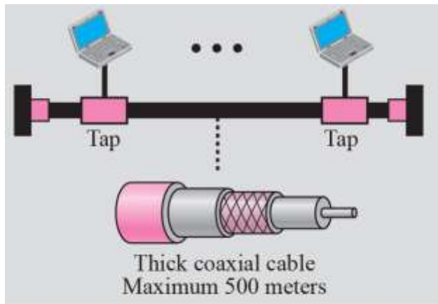
a. 10BASE5
