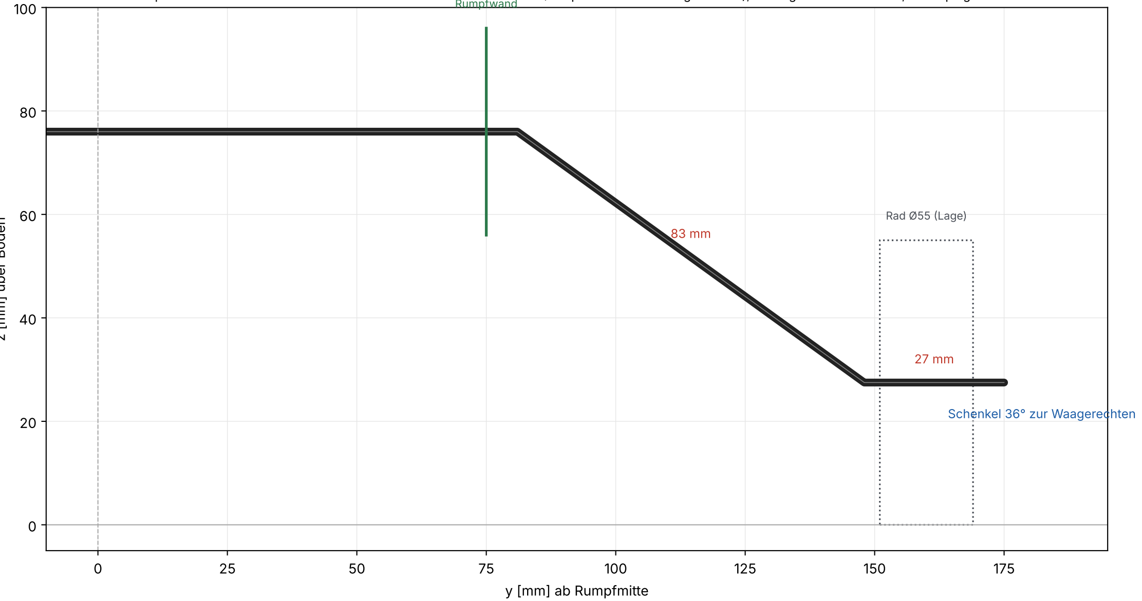
Hauptfahrwerk: Federstahldraht Ø4 mm - rechte Hälfte im Maßstab 1:1 (A4 quer ohne Skalierung drucken), Draht gesamt ca. 391 mm, links spiegeltbildlich
