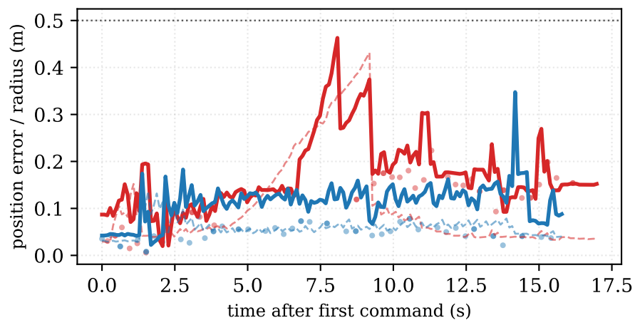
(d) Truth-belief error with 2\sigma belief radius
