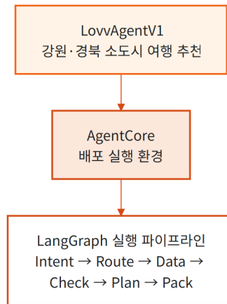
LowAgentV1 실행 구조
