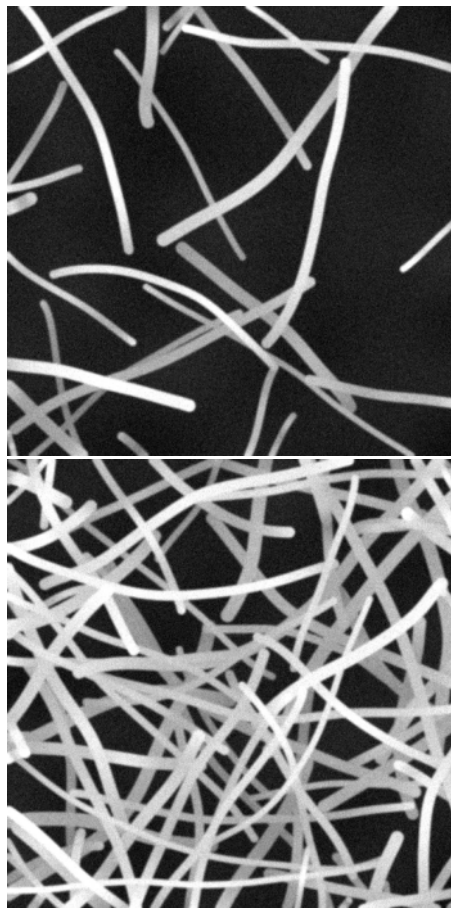
Synthetic SEM
