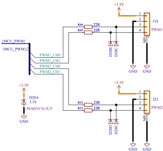
PWM
