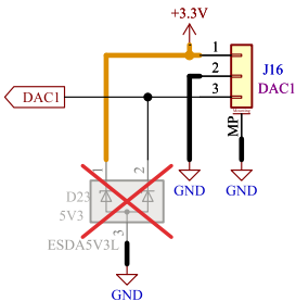
DAC
