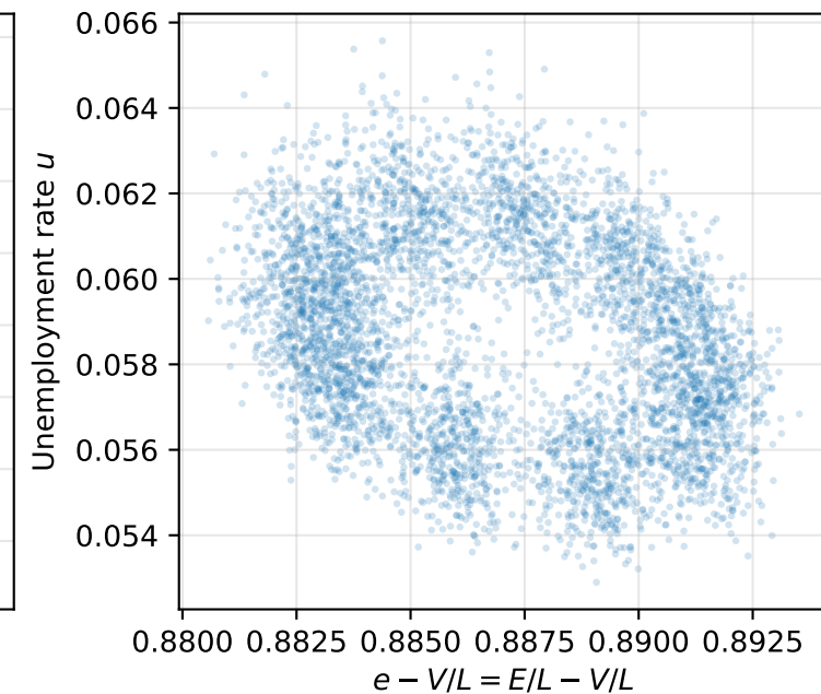
u vs e - V/L
