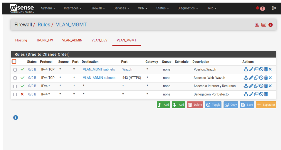
Figura 10. WebGUI FW-Interno – reglas interfaz VLAN_MGMT.
