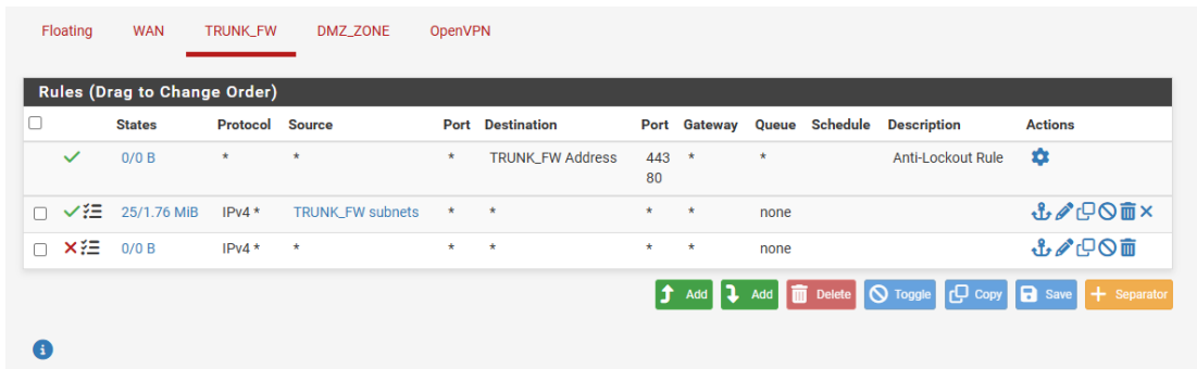
Figura 6. WebGUI FW-Externo – reglas interfaz TRUNK_FW.
