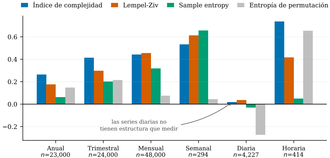
Correlación con el sMAPE del Naive
