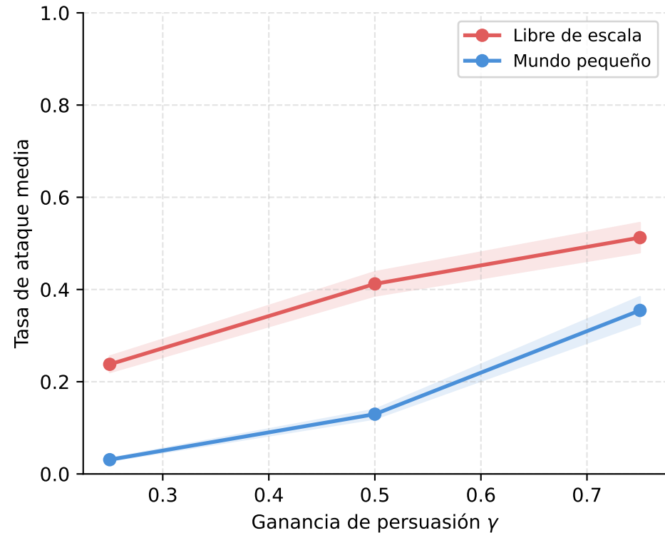
Sensibilidad de la tasa de ataque a los factores de mayor impacto
