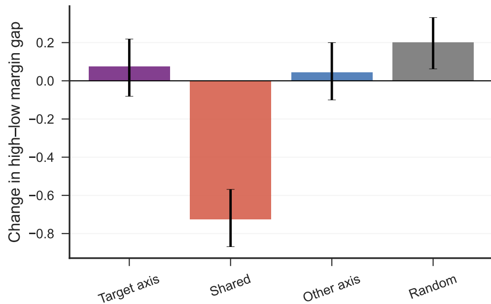
Gemma-3-27B — Warmth
