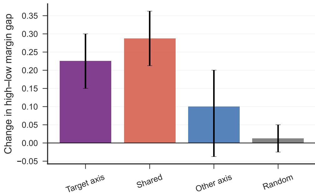
Gemma-3-12B — Warmth
