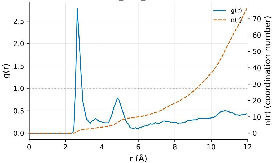
rdf_OD1_water
