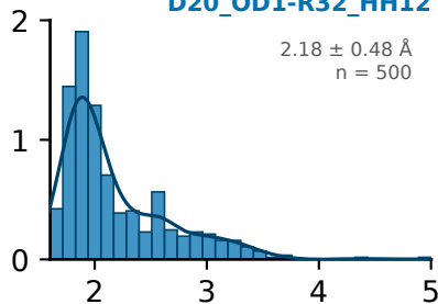
D20_OD1-R32_HH12
