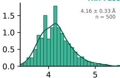
TRH-F255
