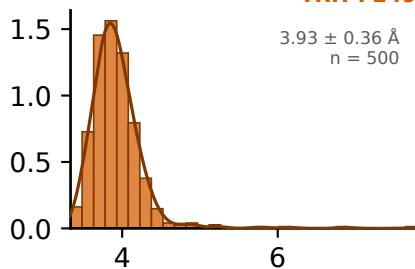
TRH-F249
