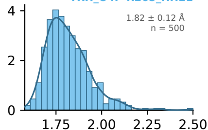
TRH_O4P-R265_HH21
