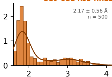
D20_OD2-R32_HH22
