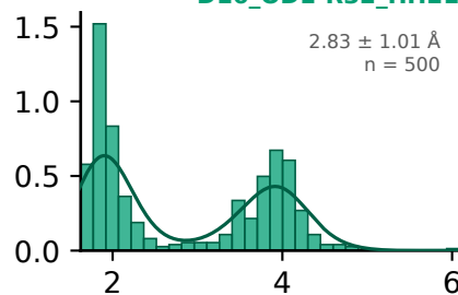
D16_OD1-R32_HH21
