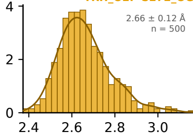
TRH_O2P-S272_OG
