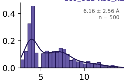
E89_OE2-K55_NZ
