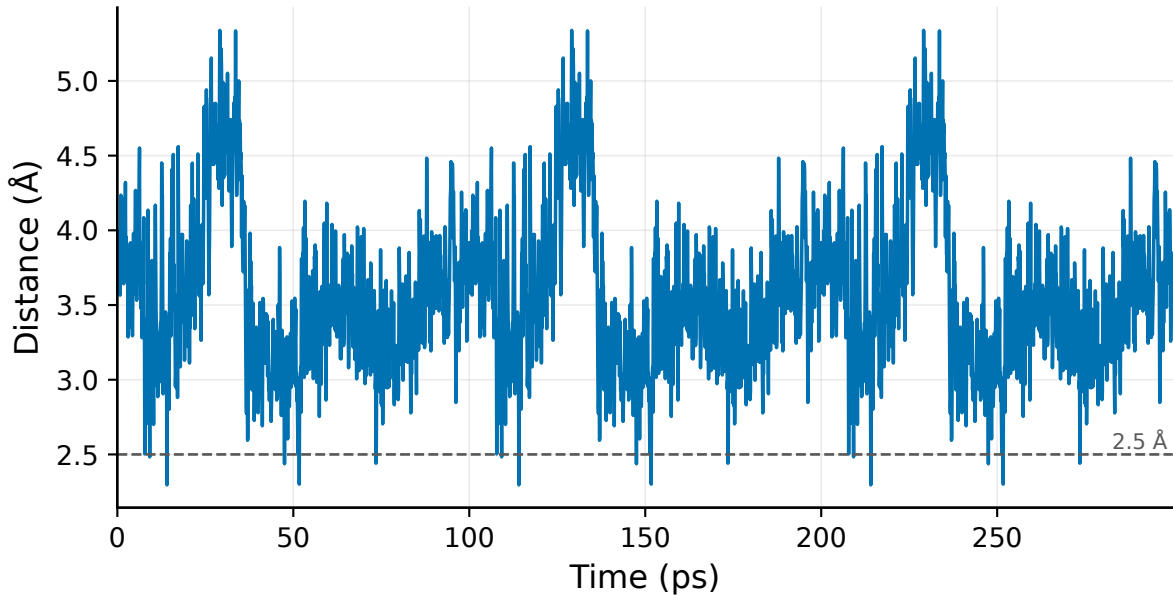
d_TRH_O4P_R268HH21
