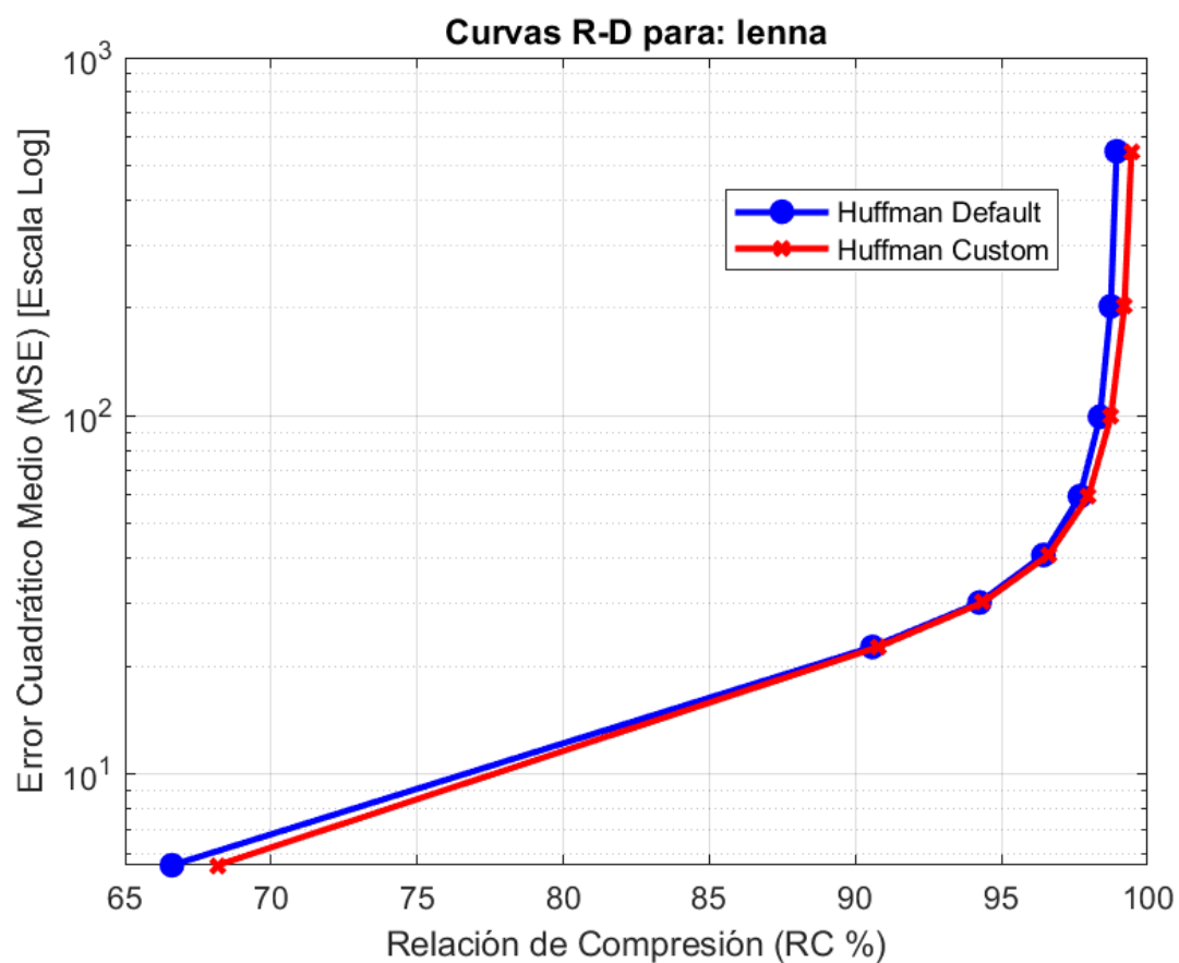
Figura 13: lenna: MSE vs RC ( %) en Escala Semilogarítmica.
