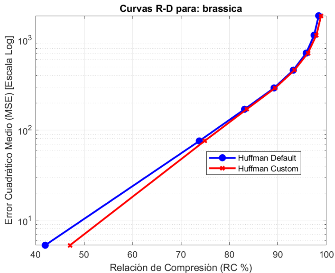
Figura 25: brassica: MSE vs RC ( %) en Escala Semilogarítmica.
