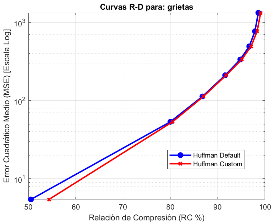
Figura 22: grietas: MSE vs RC ( %) en Escala Semilogarítmica.
