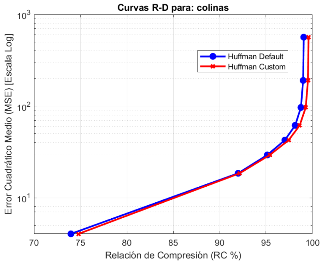
Figura 28: colinas: MSE vs RC (%) en Escala Semilogarítmica.
