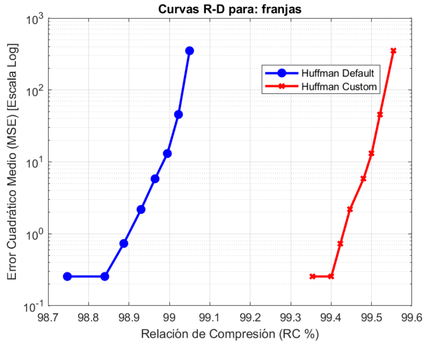
Figura 10: Franjas: MSE vs RC (%) en Escala Semilogarítmica.
