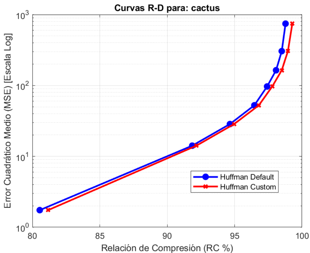
Figura 19: cactus: MSE vs RC ( %) en Escala Semilogarítmica.
