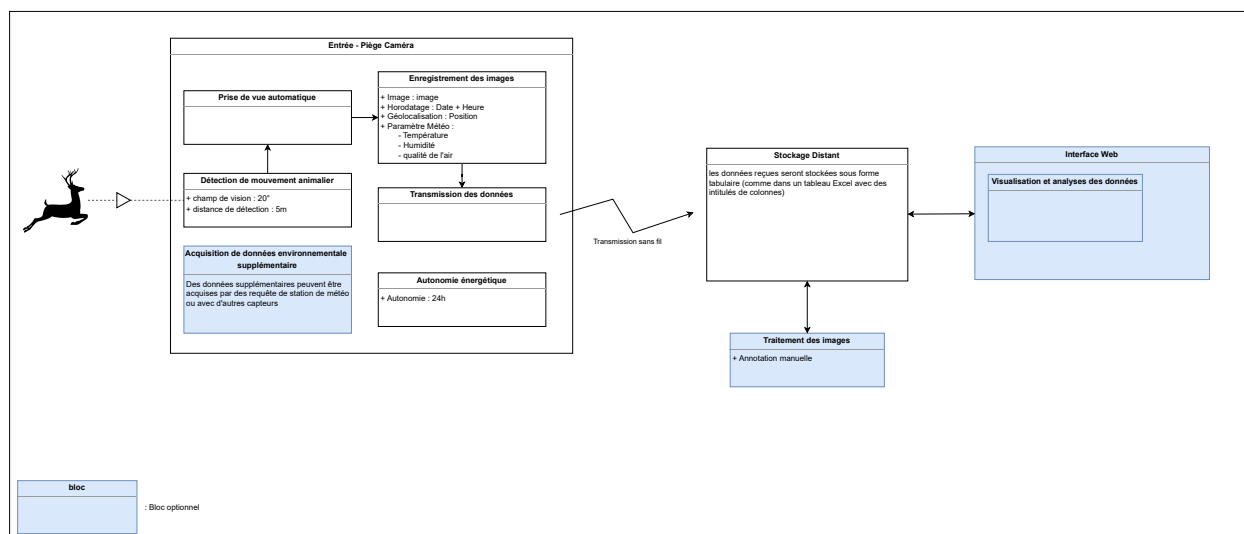
FIGURE II.3 – Décomposition en bloc fonctionnel principale et optionnelle
