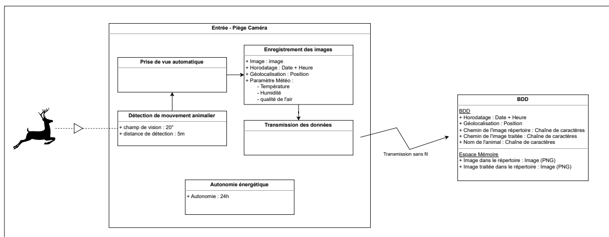
FIGURE X.2 – Décomposition en bloc fonctionnel principale
