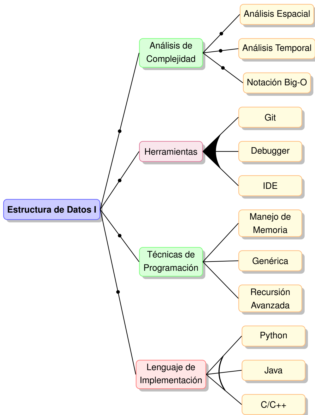
Figura 3: Representación simplificada #2 del FM de la asignatura Estructura de Datos I. Fuente: elaboración propia.
