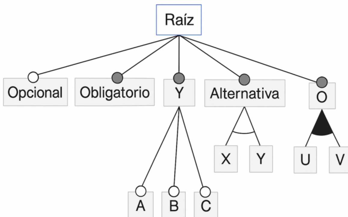
Figura 1: Símbolos gráficos para representar las relaciones estructurales. Fuente: Elaboración propia.
