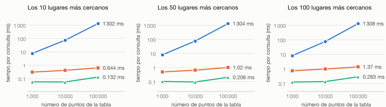
Figura 5: Vecinos más cercanos. El R-Tree y GiST son casi planos: su coste apenas depende del tamaño de la tabla.
