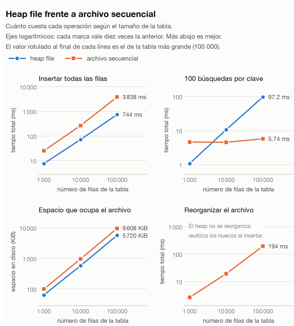
Figura 2: Heap file frente a archivo secuencial. En la búsqueda se ve el cruce: el heap sube en diagonal y el secuencial es casi plano.
