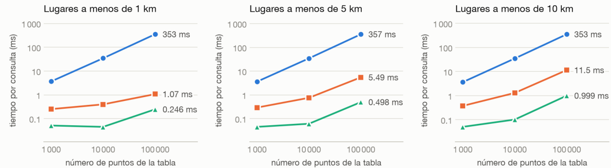
Figura 4: Consultas por radio. La línea del recorrido secuencial es la misma en los tres paneles: no depende del radio.
