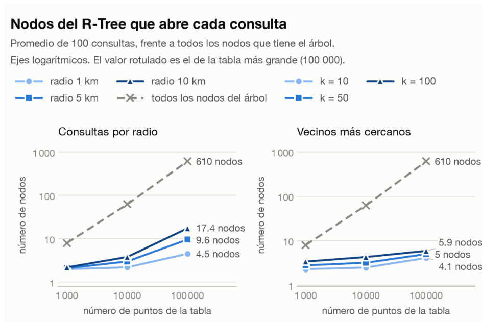
Figura 6: Nodos del R-Tree que abre de media cada consulta, frente a todos los que tiene el árbol (línea gris discontinua).
