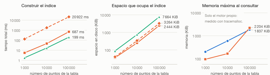
Figura 7: Construir el índice, guardarlo y consultarlo. La línea discontinua es el mismo R-Tree construido insertando los puntos de uno en uno en vez de con carga masiva.
