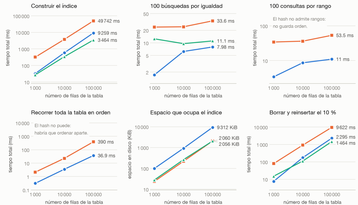
Figura 3: B+ agrupado, B+ no agrupado y hash extendible. En el rango y en el recorrido ordenado falta la línea del hash: no puede hacer ninguna de las dos cosas.
