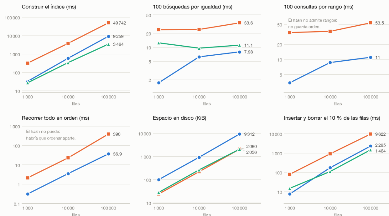
Figura 2: B+ agrupado, B+ no agrupado y hash extensible. En rango y recorrido ordenado falta la línea del hash: no puede hacer ninguna de las dos cosas.
