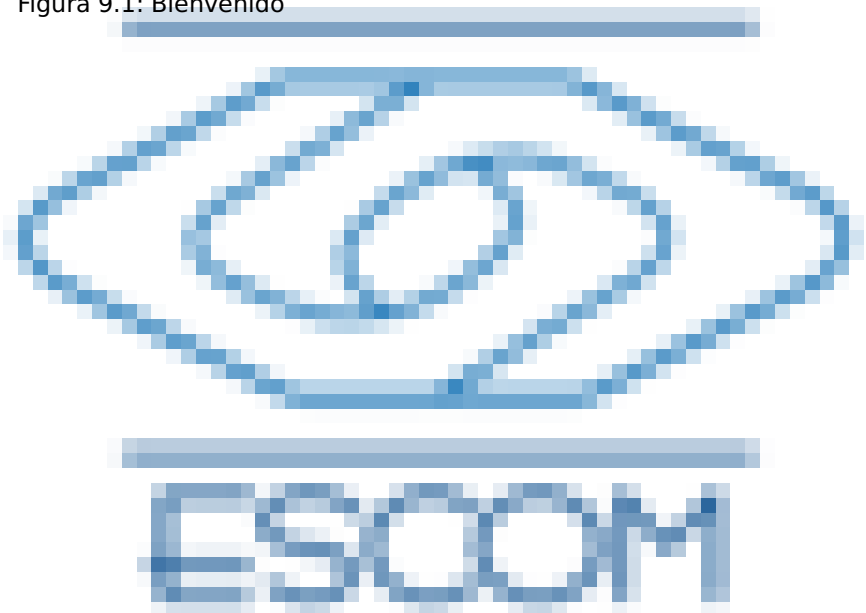
Figura 9.1: Bienvenido
