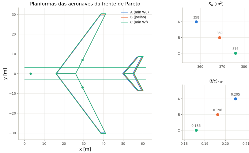
Figura 6: Planformas das três aeronaves selecionadas.
