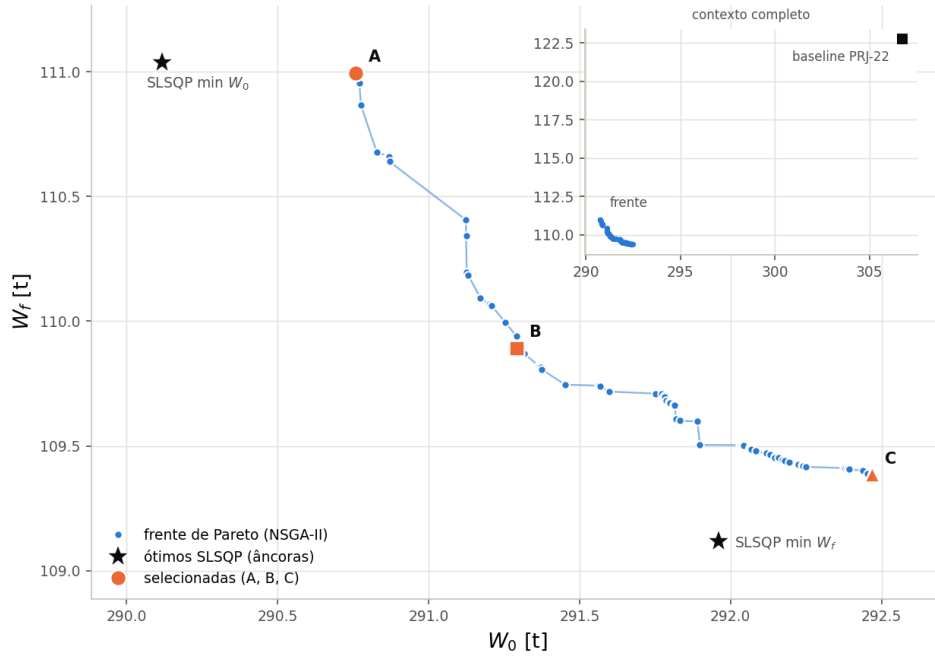
Figura 5: Frente de Pareto W_0 \times W_f , com a baseline, os ótimos mono-objetivo (SLSQP) e as três aeronaves selecionadas.
