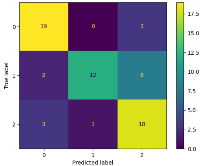
Figura 11: Matriz de confusión del test sobre el test del modelo
