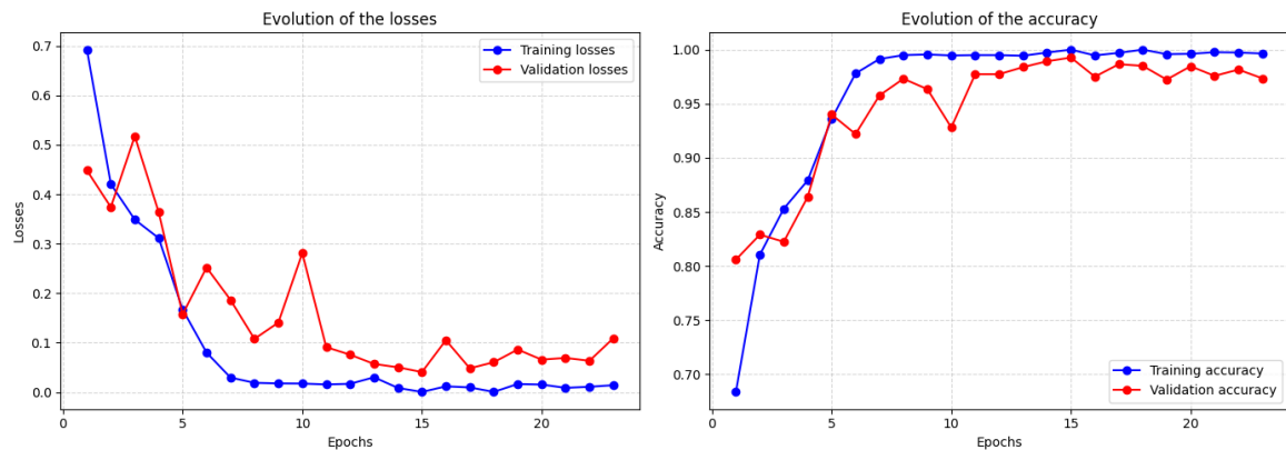
Figura 10: Resultados de un entrenamiento con la evolución de las pérdidas a la izquierda, y de la eficiencia a la derecha
