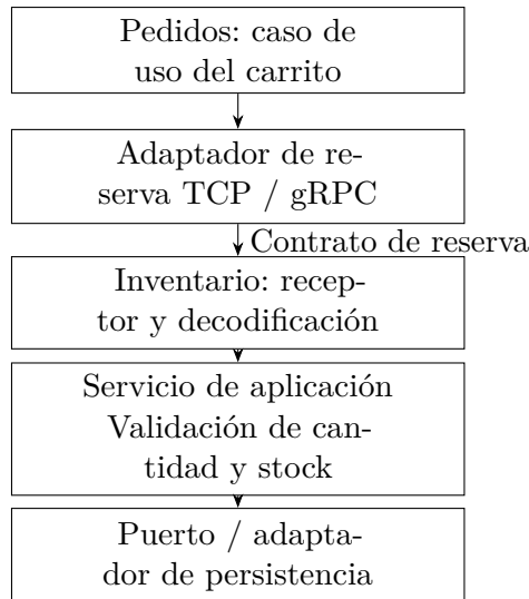
Figura 3: C4 nivel 3: componentes del recorrido de reserva; vista propia de responsabilidades.
