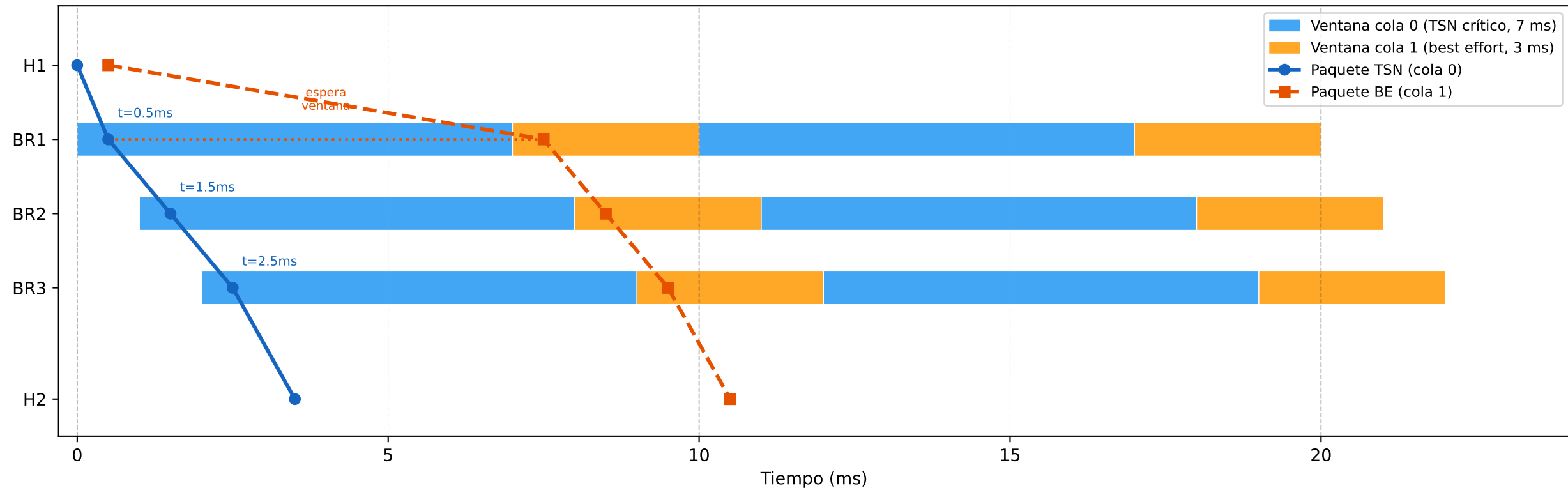
Flujo de paquete TSN vs. best-effort — cadena BR1→BR2→BR3
