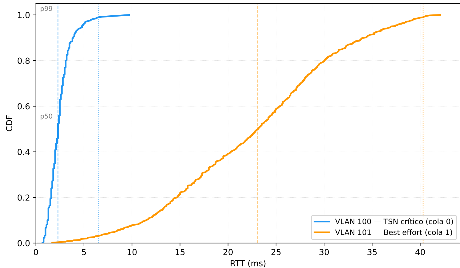
CDF de latencia RTT — TSN crítico vs. best effort
